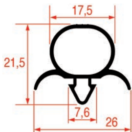
PROFIL A ENCASTRER - 1032
