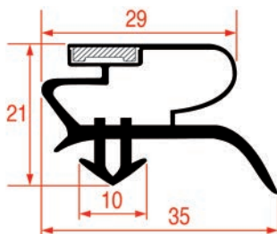
PROFIL A ENCASTRER - 1053
