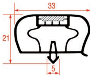
PROFIL A ENCASTRER - 1051
