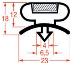
PROFIL A ENCASTRER - 9199
