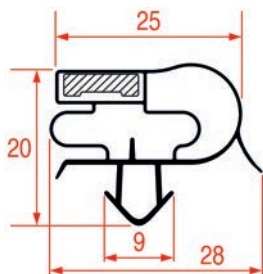
PROFIL A ENCASTRER - 1078
