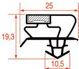
PROFIL A ENCASTRER - 1035
