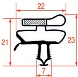
PROFIL A ENCASTRER - 1088
