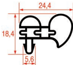
PROFIL A ENCASTRER - 1027
