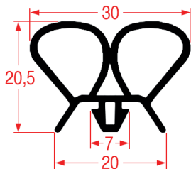
PROFIL A ENCASTRER - 9938
