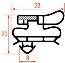
PROFIL A ENCASTRER - 1052
