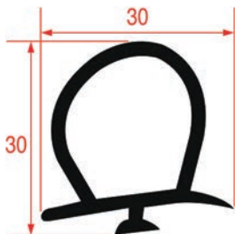
PROFIL JOINT DE CELLULE - 9994
