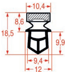
PROFIL A ENCASTRER - 9325
